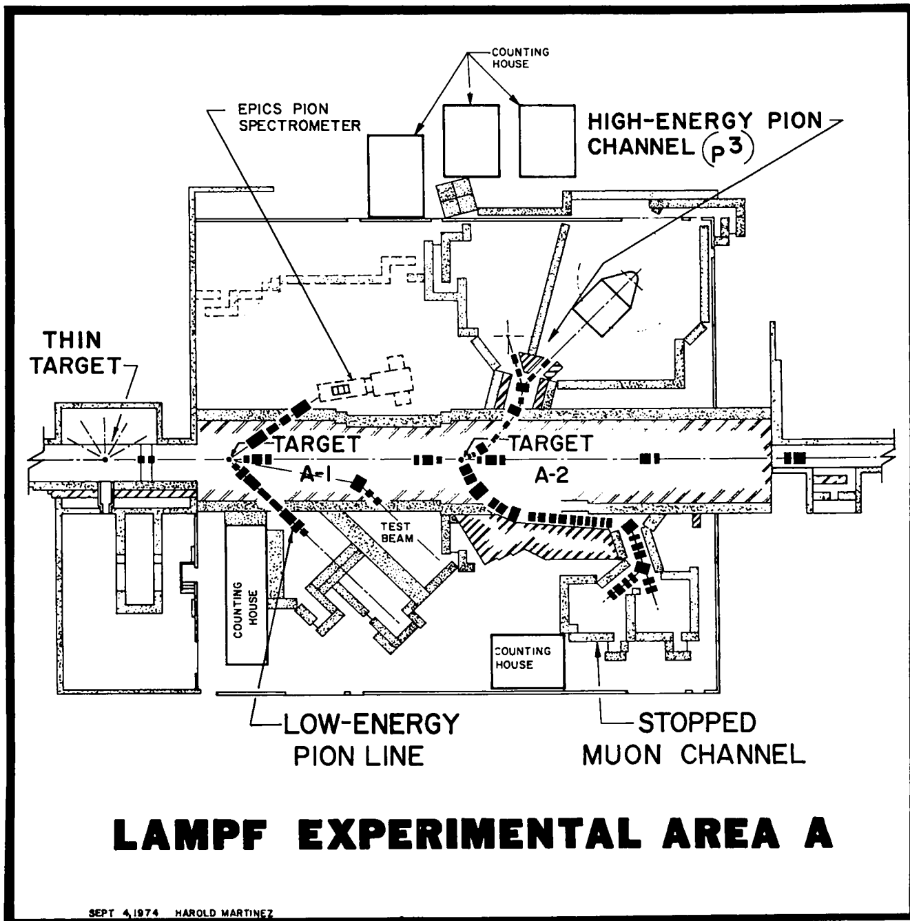
Fig. 13. Experimental Area A.
