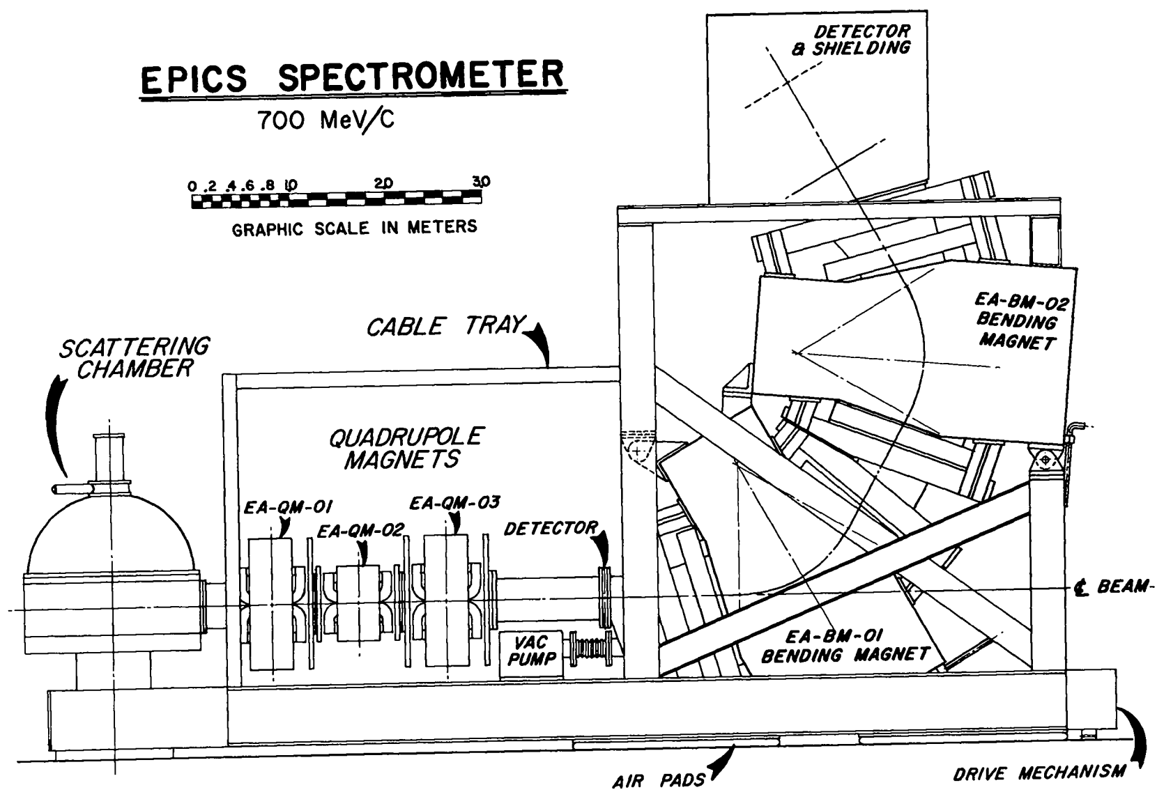
Fig. 17. EPICS Spectrometer.
